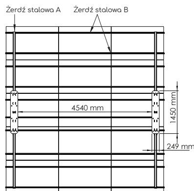
Przekrój - widok z dołu
