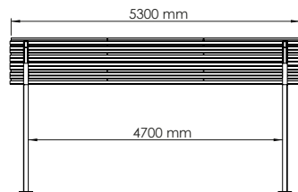
Przekrój - widok z przodu
