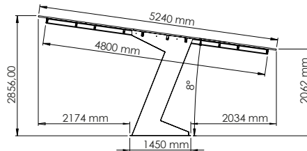
Przekrój - widok z boku
